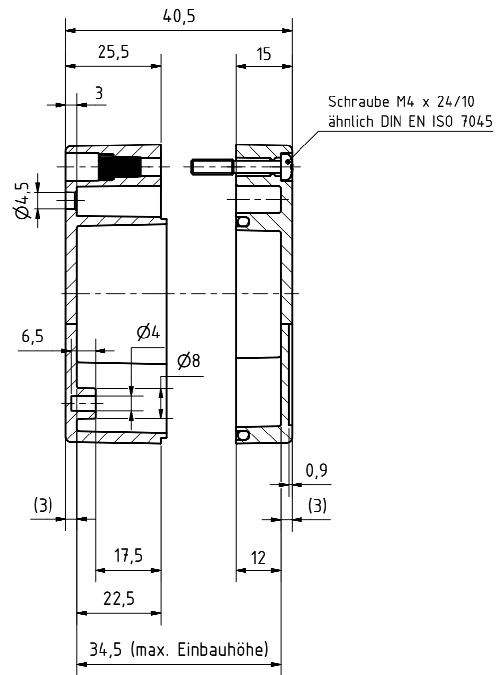
A-A ( 1 : 1 )
